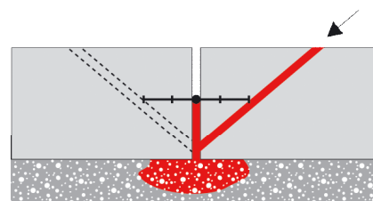
Fig. 5: Etanchement des joints de dilatation à posteriori
