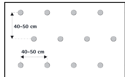
Fig. 2: Disposition et maillage standard des forures pour l'étanchéification de surfaces murales
