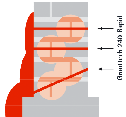
Fig. 1: Principe de fonctionnement du Grouttech 240 Rapid. Le gel est injecté sous pression dans les forures jusqu'à ce qu'il arrive de l'autre côté de la maçonnerie où il forme un voile d'étanchéité. Sur son parcours, le produit pénètre simultanément dans les joints de la maçonnerie dont il renforce l'étanchéité.
